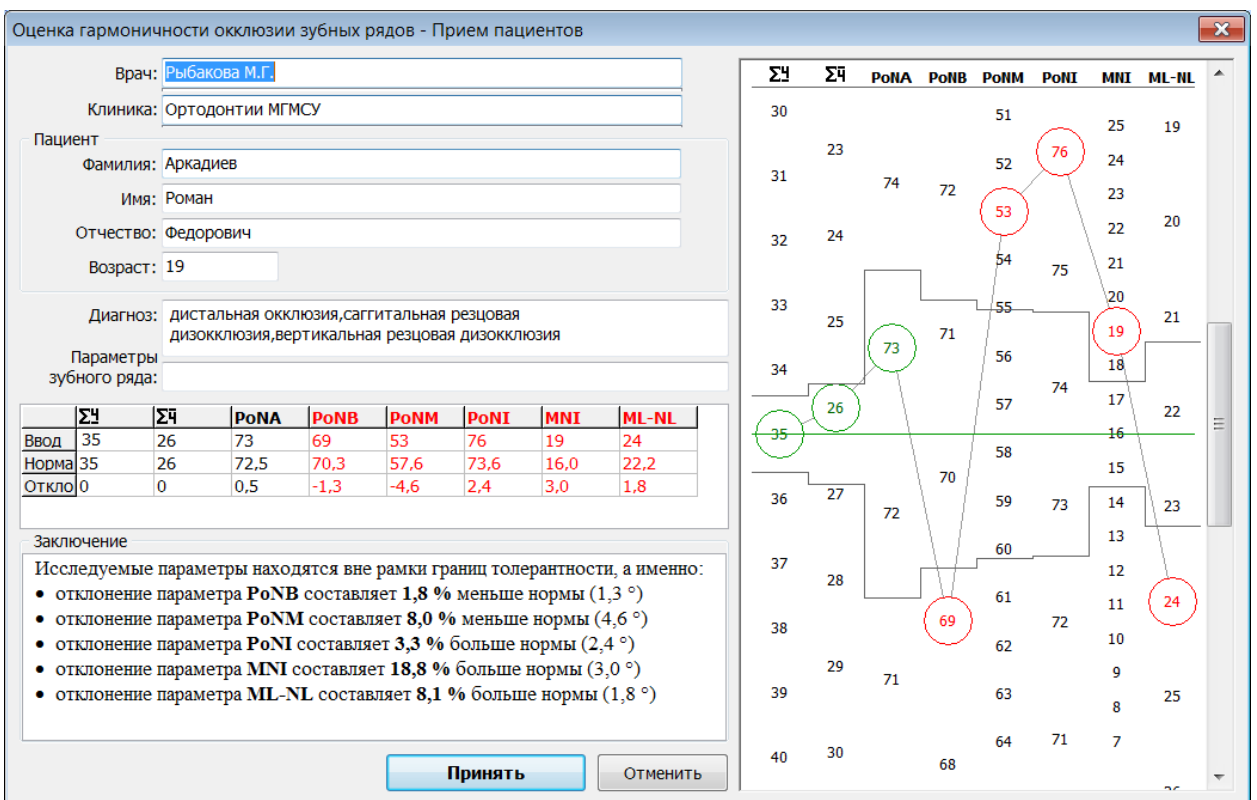
Рис.2. Рабочая страница программы
