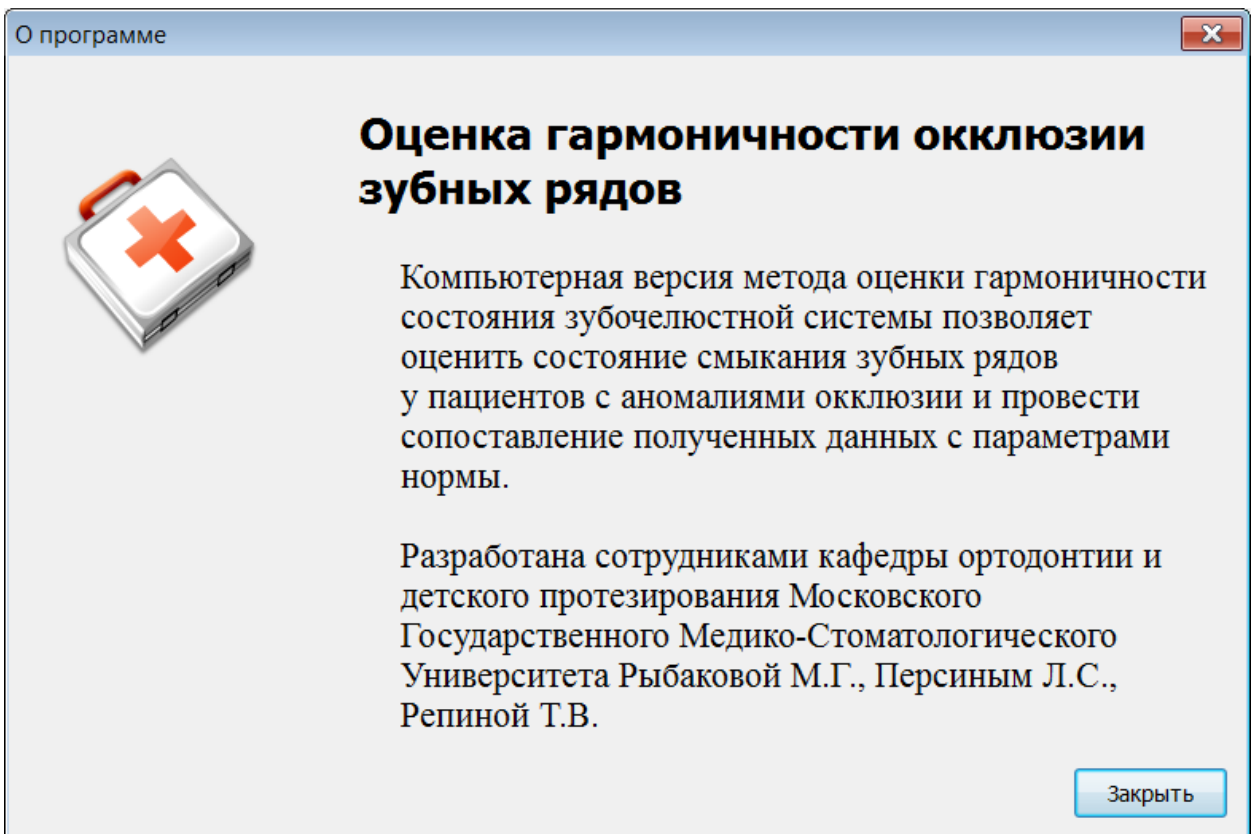
Рис.1. Интерфейс программы
